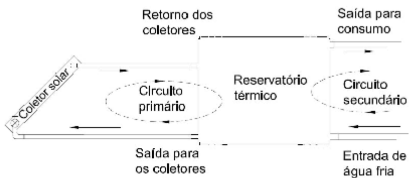
Figura 7 — A1- Esquema do SAS
