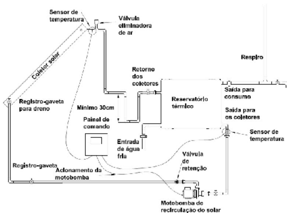
Figura 2 — Esquema de circuito para circulação forçada
