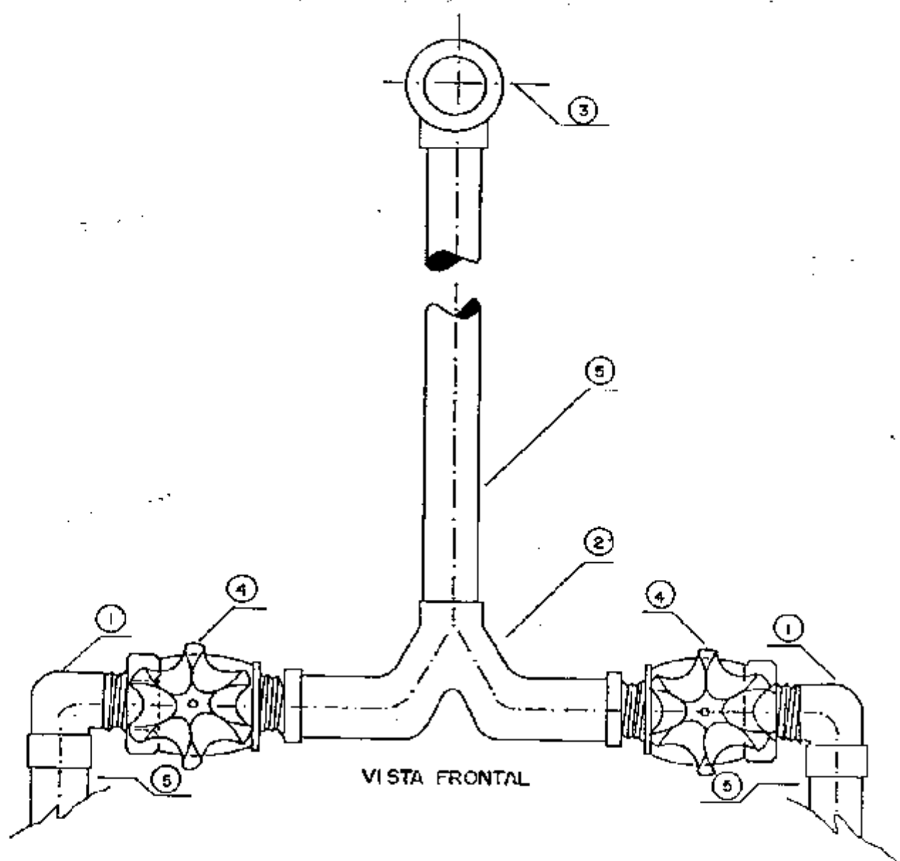
DET - MISTURADOR CHUVEIRO - A. QUENTE E/A. FRIA
