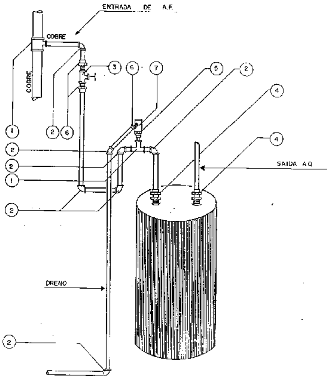
DETALHE DE INSTALAÇÃO
